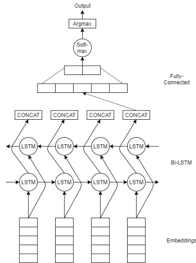
FIG. 3: Architecture du modèle de classification
