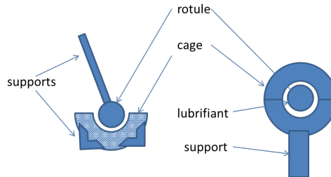
FIG. 1 – exemples de schéma de deux types d'articulations simples à rotule
