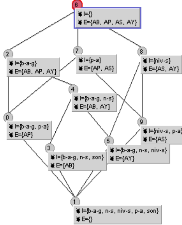
FIG. 1 – Le treillis de concepts \mathcal{L}(\mathcal{C}) correspondant au contexte formel des arrêts \mathcal{K}_{ATR} .
