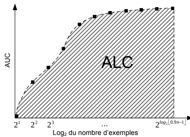
FIG. 3 – Calcul de l'ALC : aire sous la courbe d'AUC
